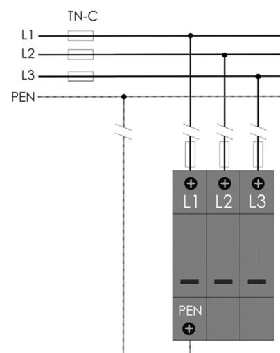
Koblingskjema
